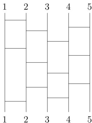
図 1: あみだくじの例
