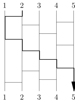
図 2: あみだくじのたどり方
